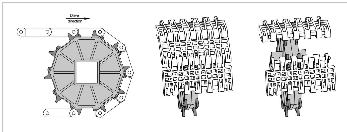
CENTRAL SPROCKET
