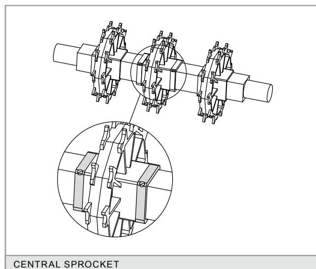
CENTRAL SPROCKET
